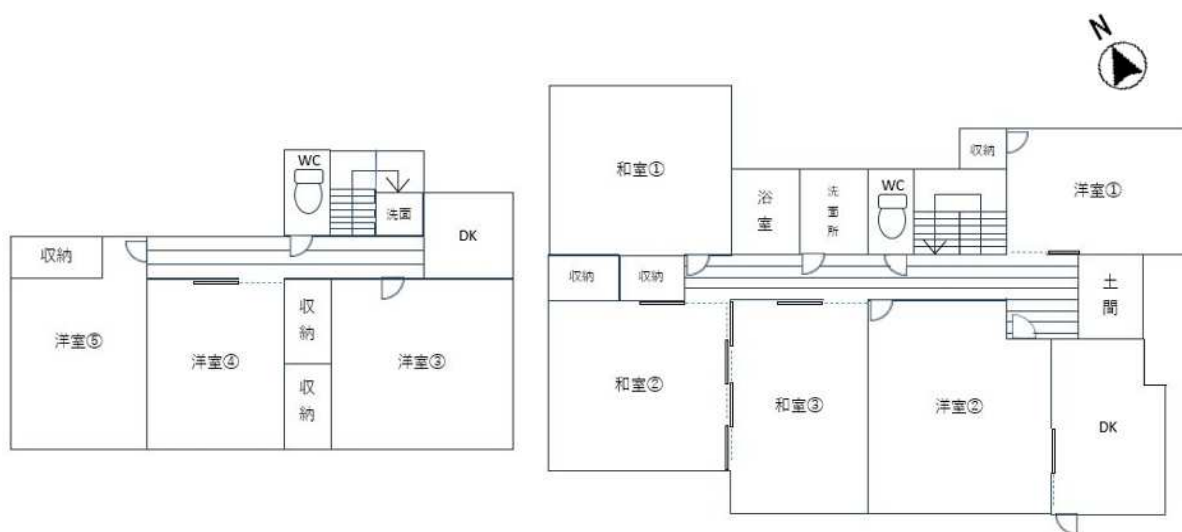
(2 階) 平面図
