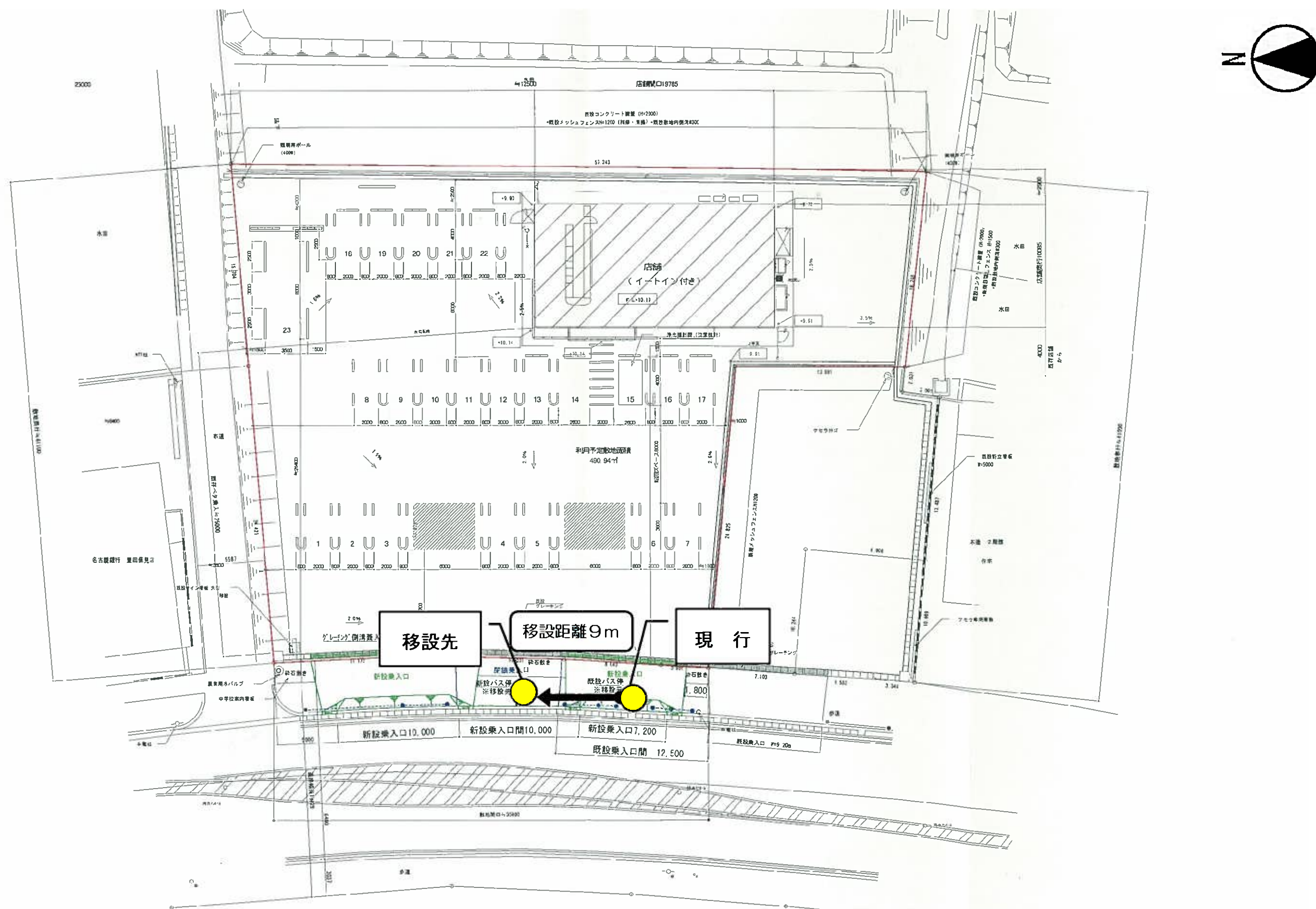
バス停移設詳細図
