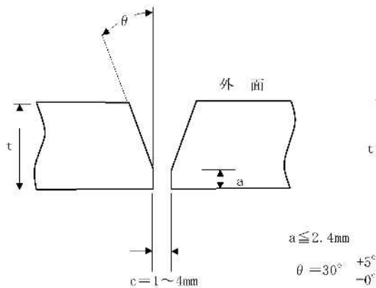
V型外開先(φ 700以下)
