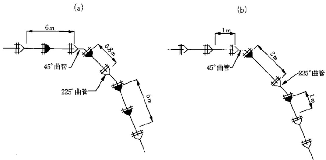
図18 複合曲管部2
