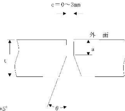
V型内開先(φ 800以上t < 16mm)
