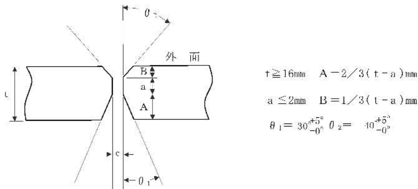
X型外開先(φ 800以上t ≥ 16mm)
