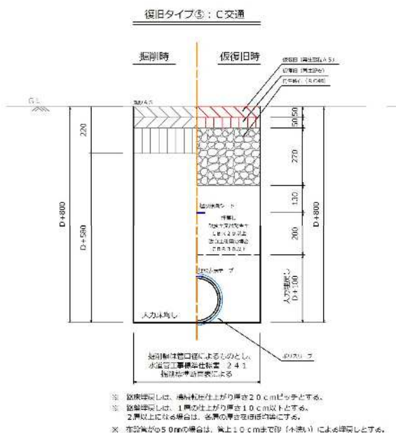
恢復旧土工標準図
