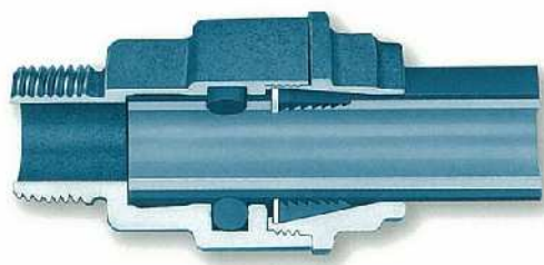
ワンタッチ式継手構造図
