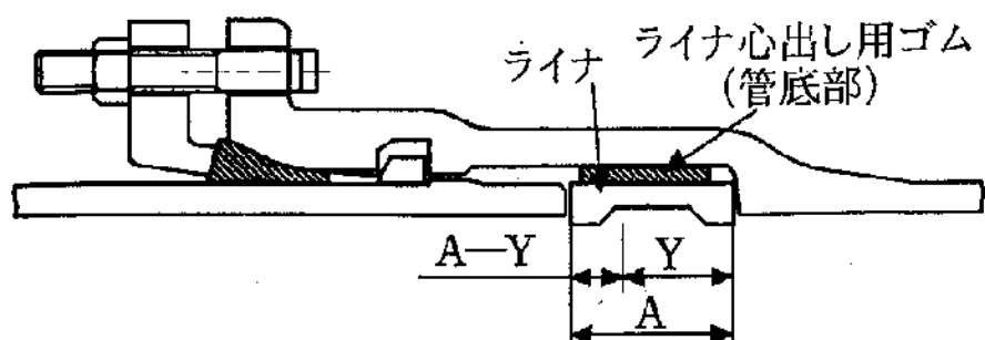
栓の継手構造（ \phi 500 mm以上）
