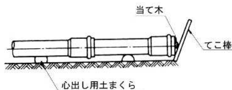
図-29 平てこ棒による挿し込み
