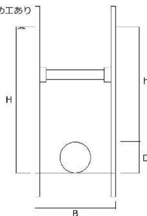
土留め工あり
