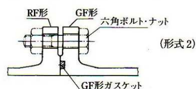
RF形—GF形の組合わせ
