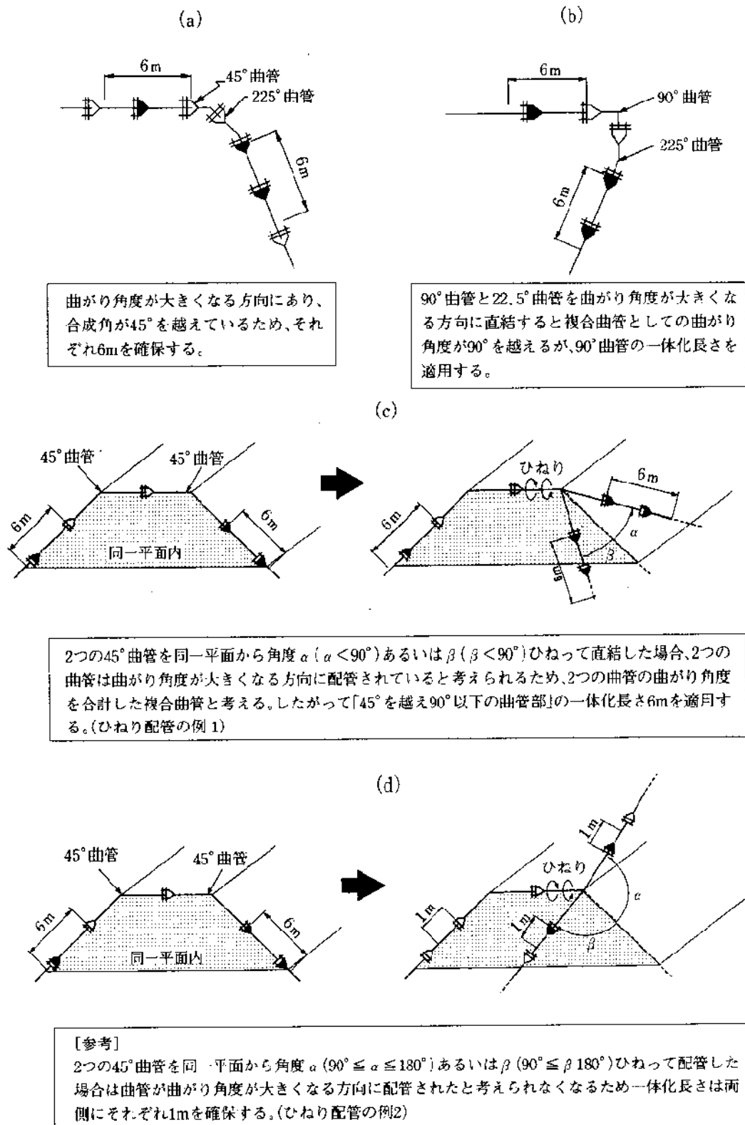
図 17 複合曲管部 1
